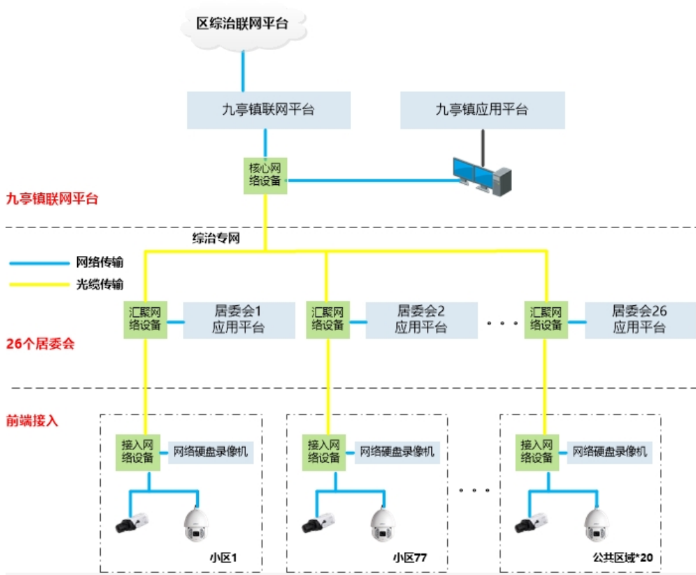
九乡镇雪亮工程系统架构图
